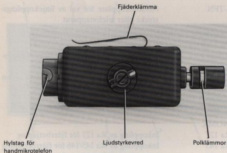
Bild 17. Linjekopplingsstycke
