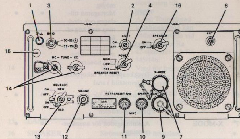
Bild 11. Ra 422, frontpanel
