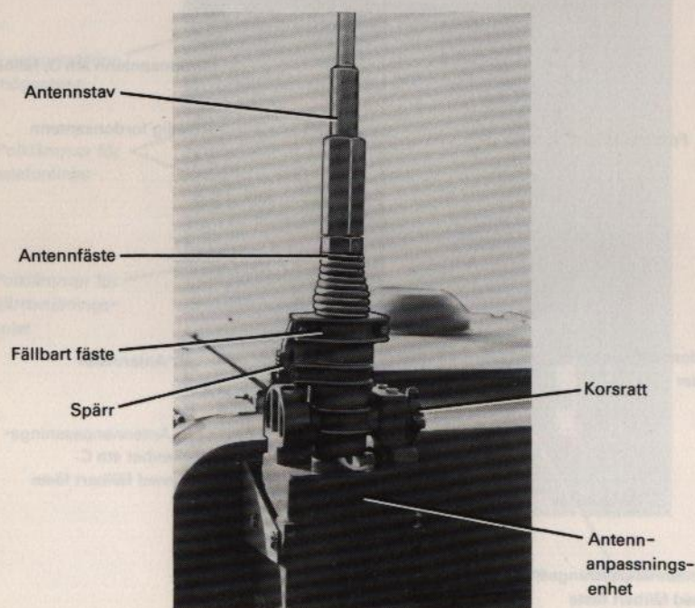
Bild 14. Antennfäste för antenn 537
