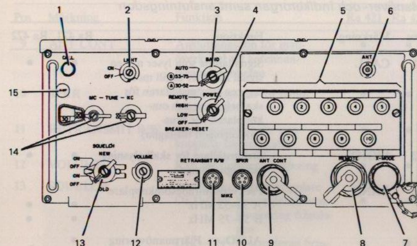
Bild 10. Ra 421, frontpanel
