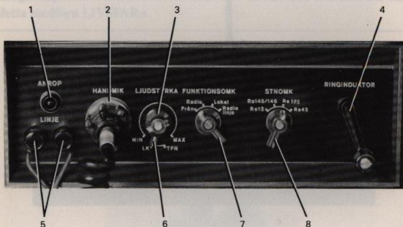
Bild 16. Fjärrbetjäningenshet, frontpanel
