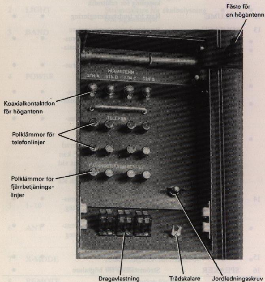
Bild 12. Yttre anslutningsfack
