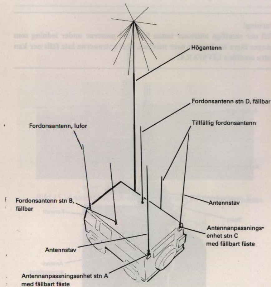
Bild 13. Antenner
