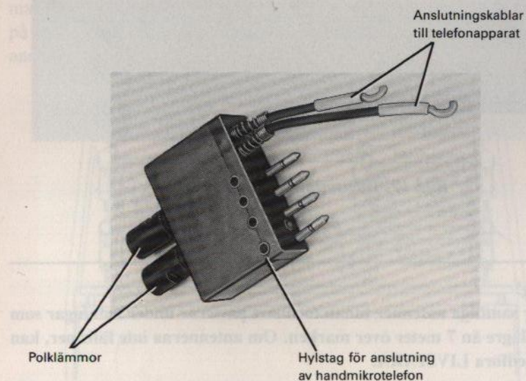
Bild 18. Mellankopplingsstycke
