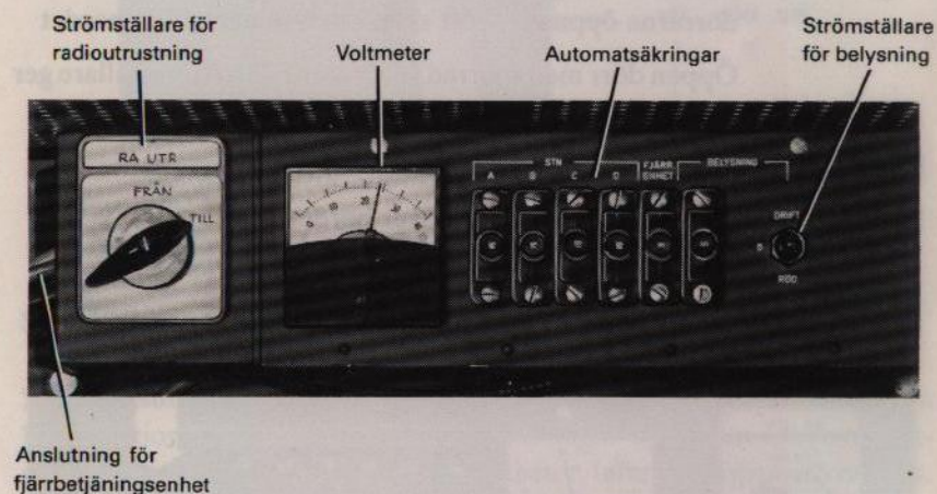
Bild 4. Strömförsörjningsenhet
